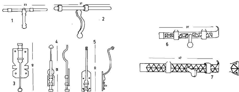
Fig. 29. Pasadores.
