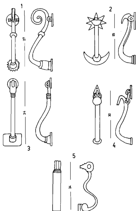
Fig. 23. Aldabas.
