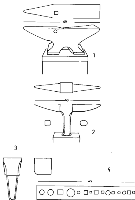
Fig. 41. Herramientas. Taller Jesús Juanto.
