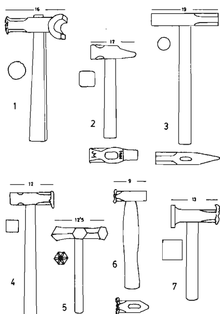
Fig. 42. Herramientas. Taller Jesús Juanto.
